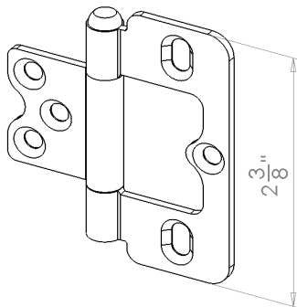
2.375" L Hinge
